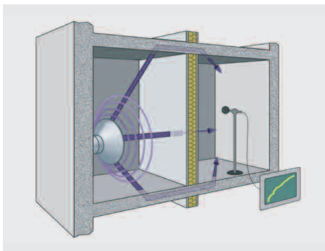
Figuur 3 Flankerend geluid.
