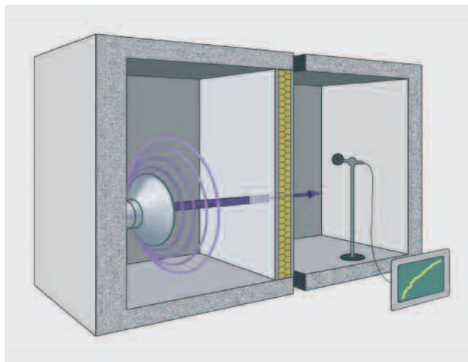
Figuur 4 Principe van ont koppeling ter verbetering van de geluidsisolatie.
